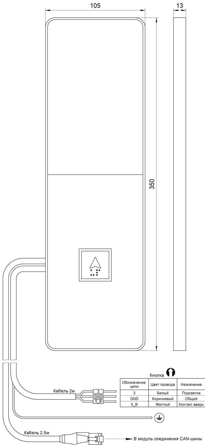
Рис.1 Внешний вид, габаритные и установочные размеры Вызывного поста МАЛАХИТ (жгут RJ45) НШЕК.468381.085
